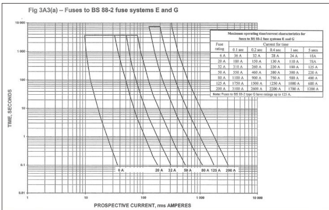
熔斷器的曲線
