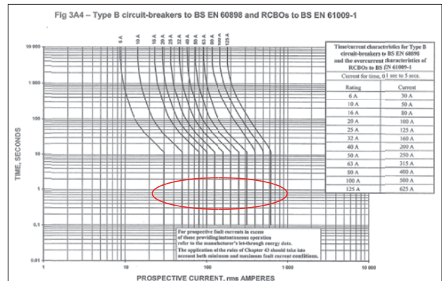
斷路器的曲線
